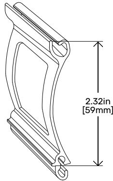
HD Bottom Bar (Optional)
